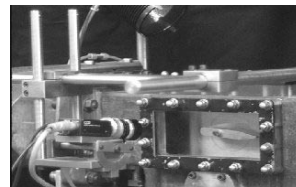
Sl. 2. Krilo in preskuševališče Fig. 2. Hydrofoil and test rig
